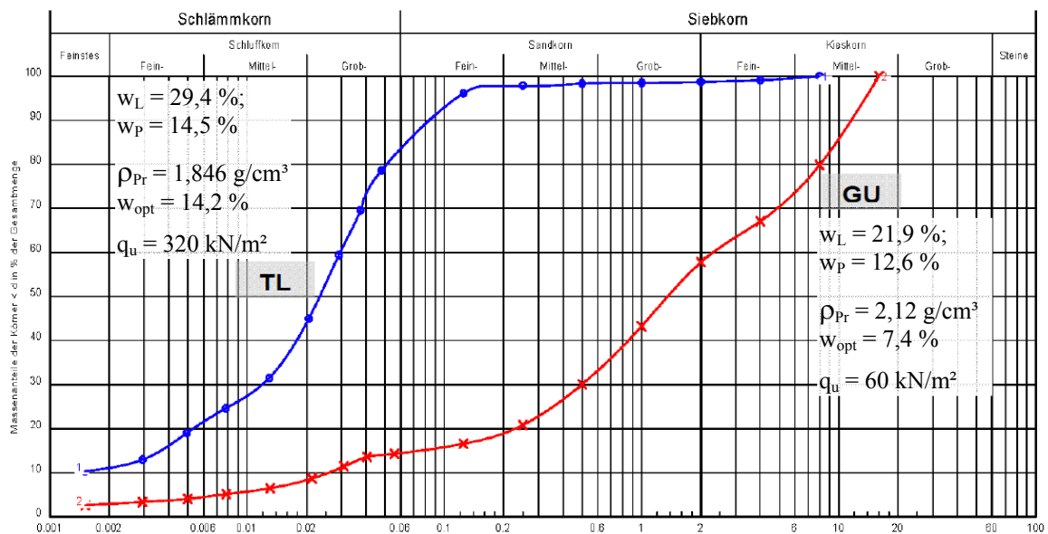
Abb. 1: Korngrößenverteilung und Charakterisierung der untersuchten Böden GU und TL [6]
